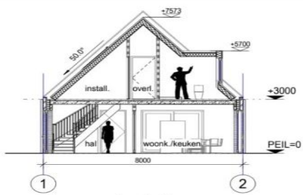
doorsnede A-A
