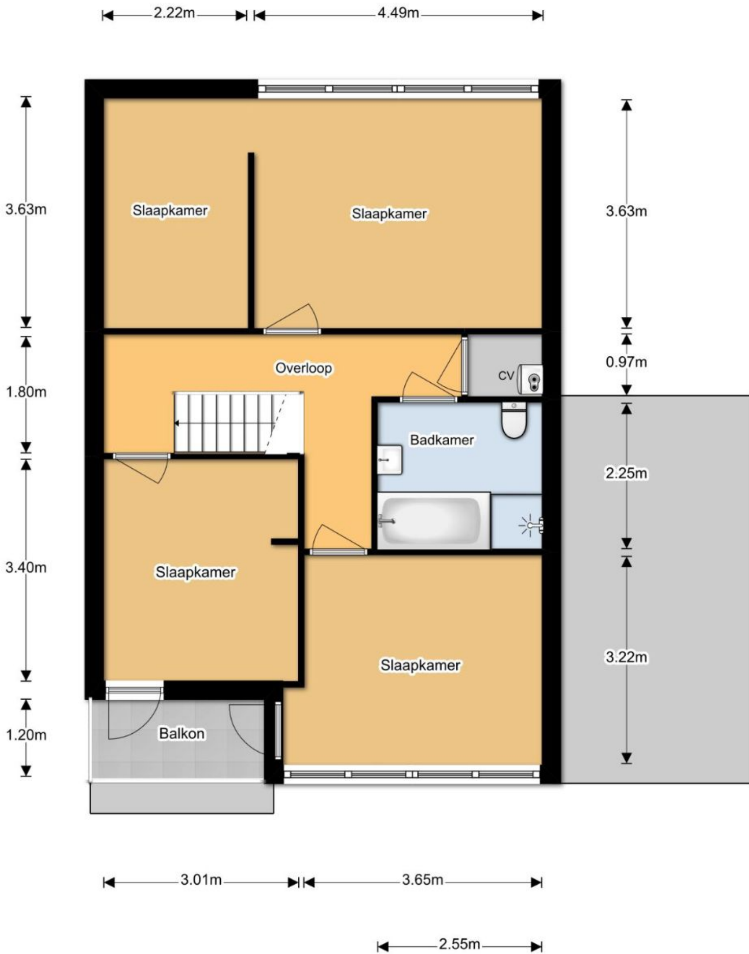
1e Verdieping
